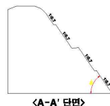
제 3 절토부 현황도 (3)
